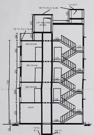
SECTION - A-B SCALE:1:100
