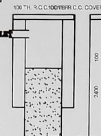
SOAKPIT.
