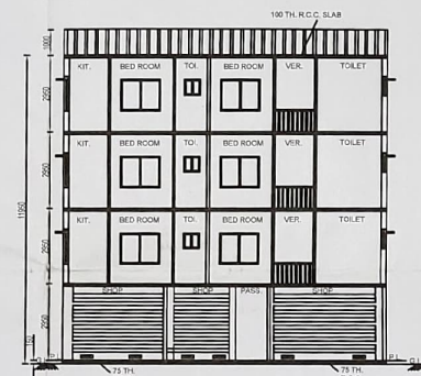
SECTION - C-D SCALE:1:100
